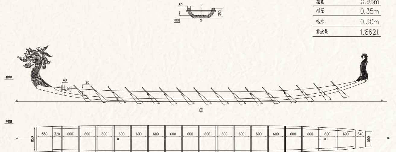
唐代独木龙舟模型设计图
