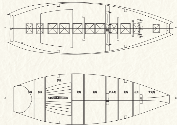
北宋海船模型设计图
